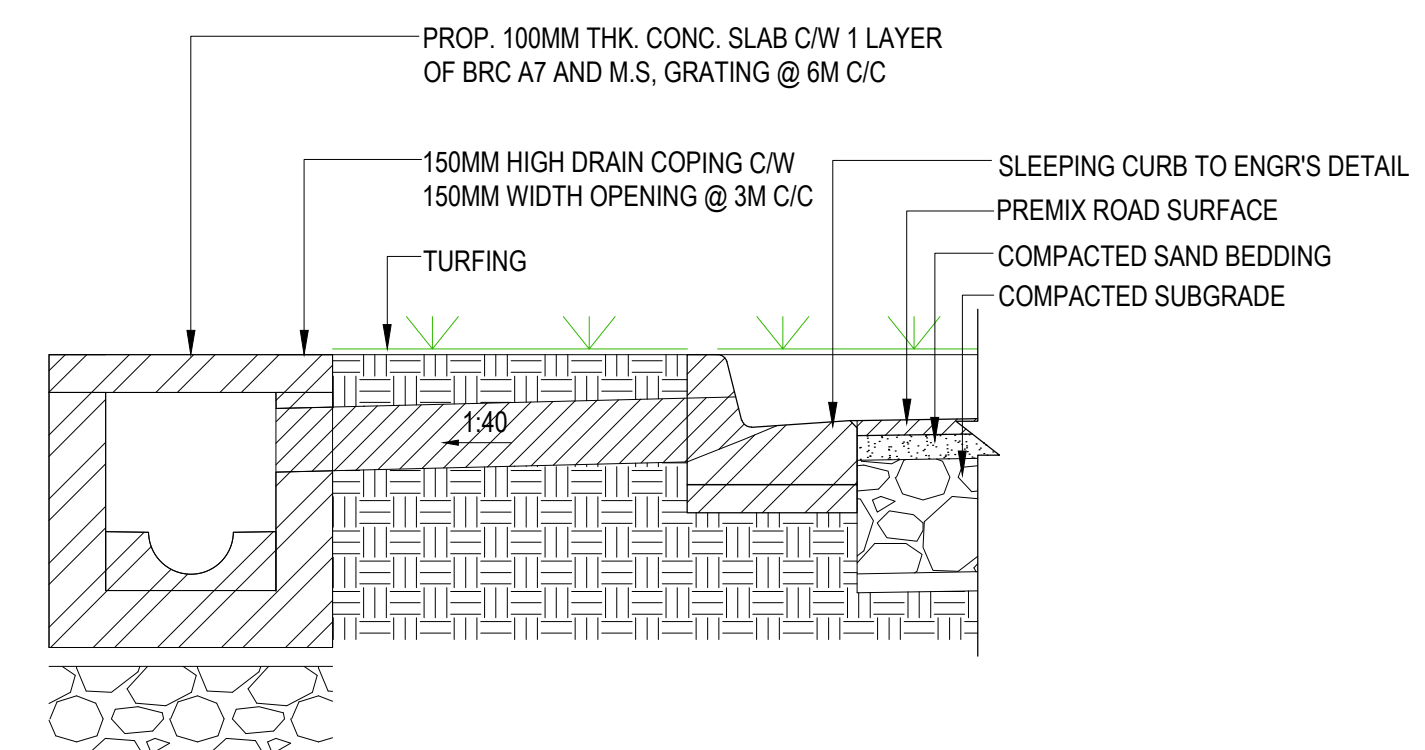
8 TIPIKAL 100mm PERINCIAN BAHU JALAN SKALA 1 : 20
