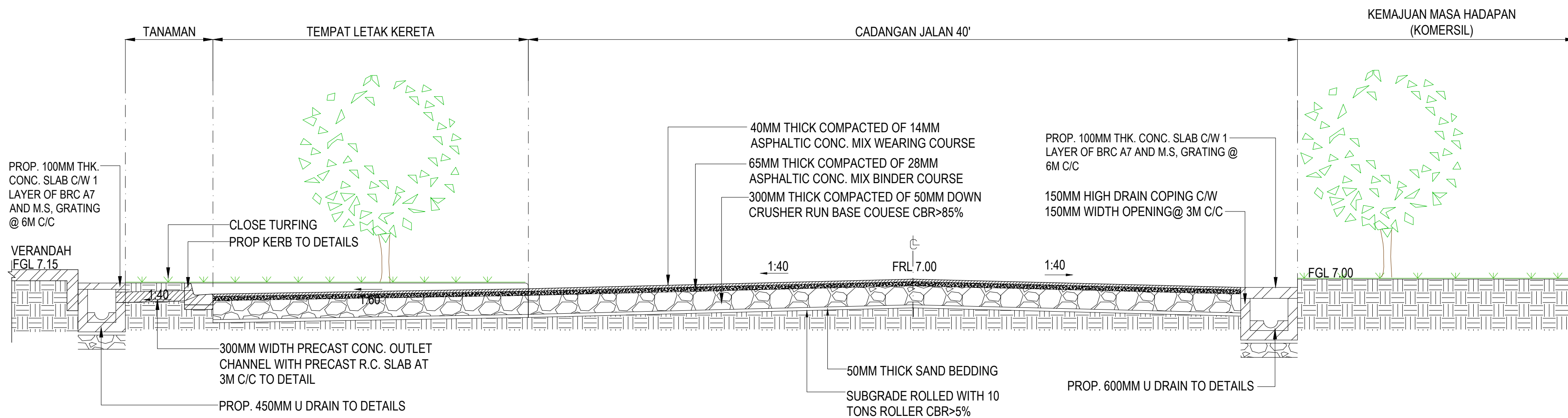
5 KERATAN E - E SKALA 1 : 50
