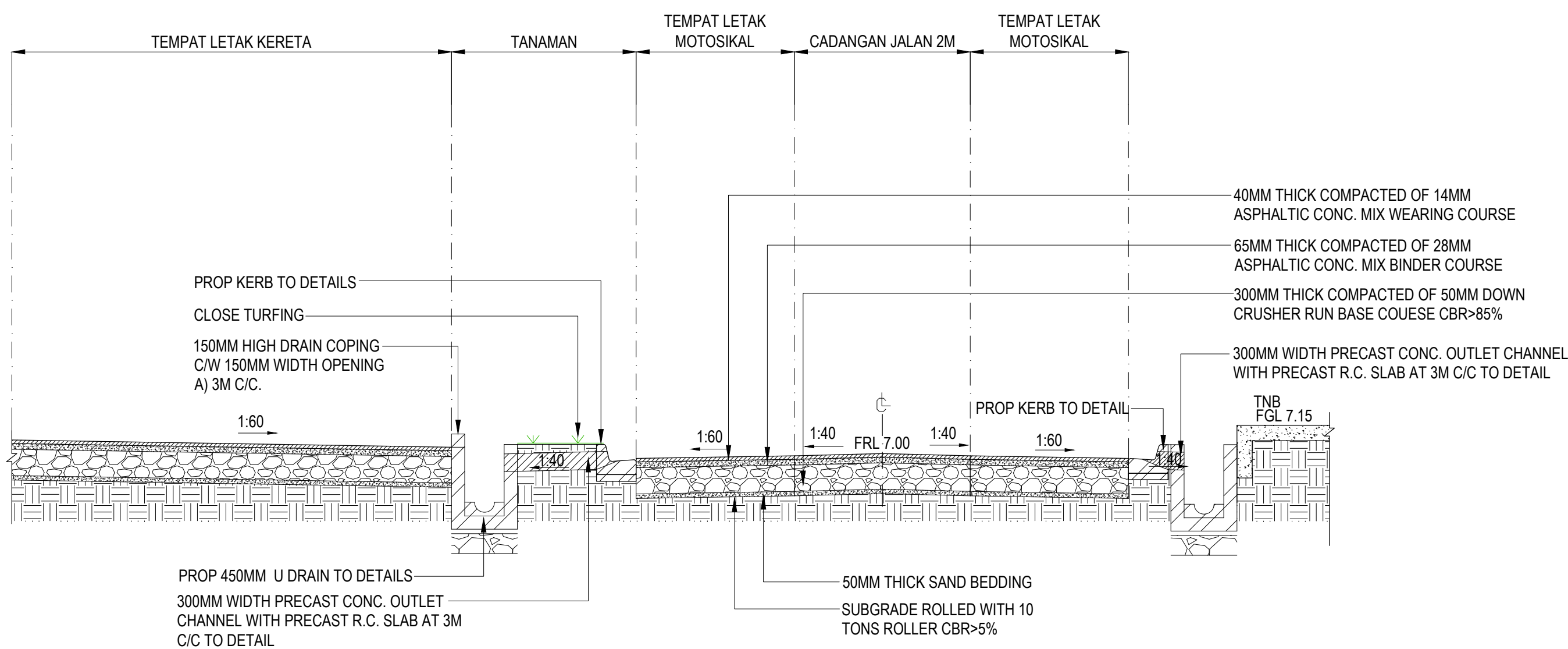
6 KERATAN F - F SKALA 1 : 50
