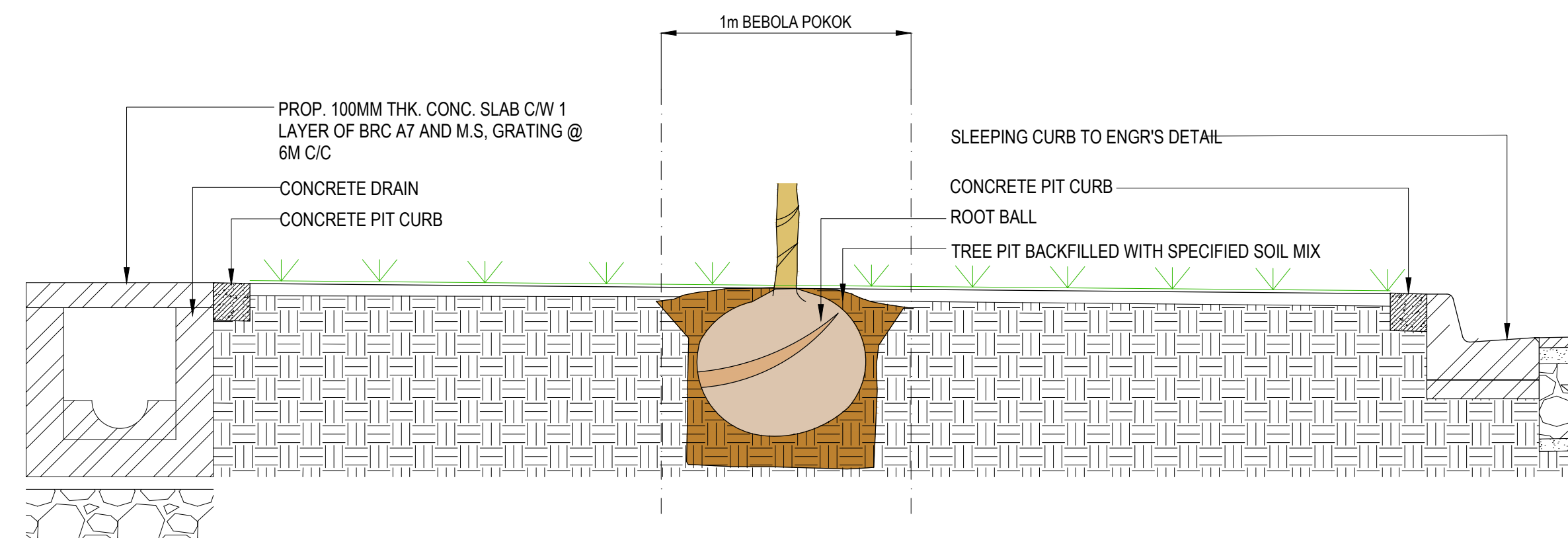
9 PERINCIAN BEBOLA POKOK SKALA 1 : 20
