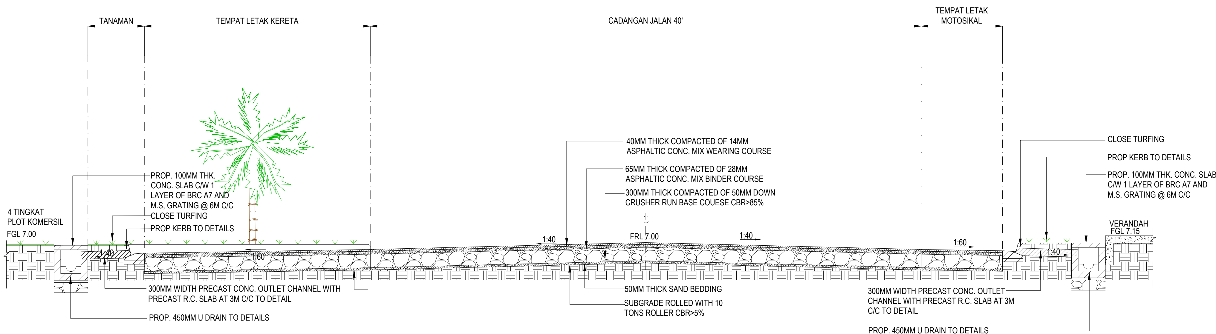
4 KERATAN D - D SKALA 1 : 50
